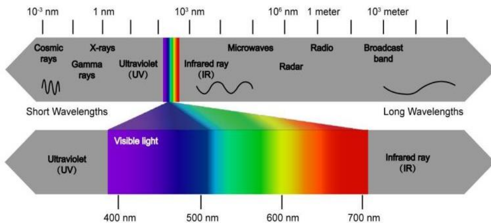
图 2.1 可见光在整个电磁波谱的位置
